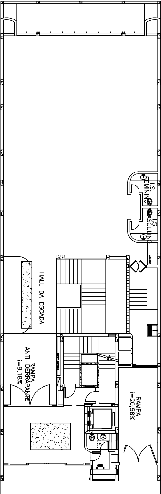
○ ESPAÇO HELIUM – SALÃO PRIMEIRO PAVIMENTO ESC. 1:175
